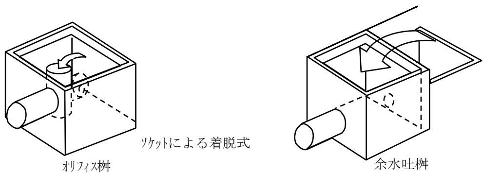
図2-8 オリフィス桷
