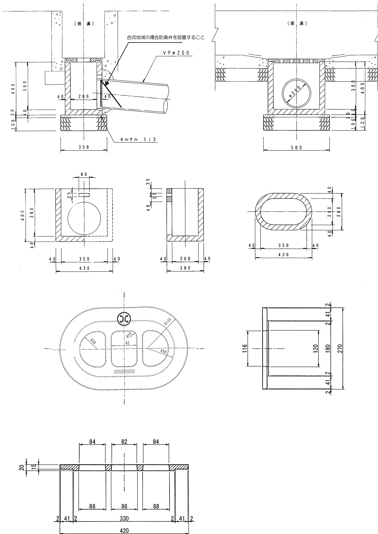
図4-4 楕円型雨水桟標準図
