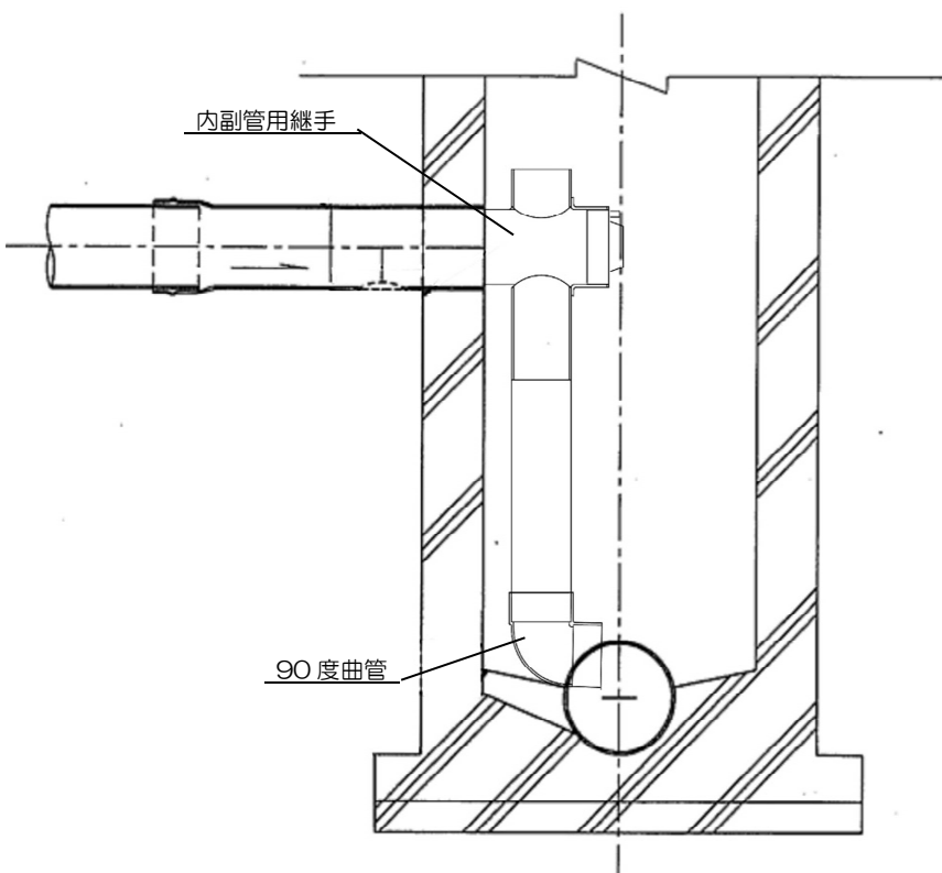
図3-7 内副管の設置例 内副管は省スペース型とする
