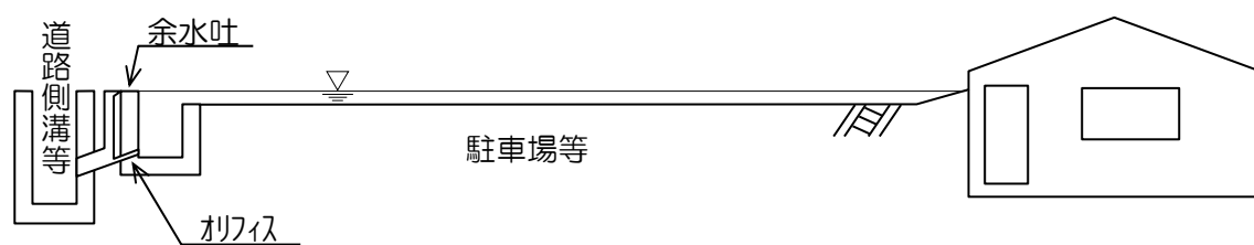
図2-4 表面貯留
