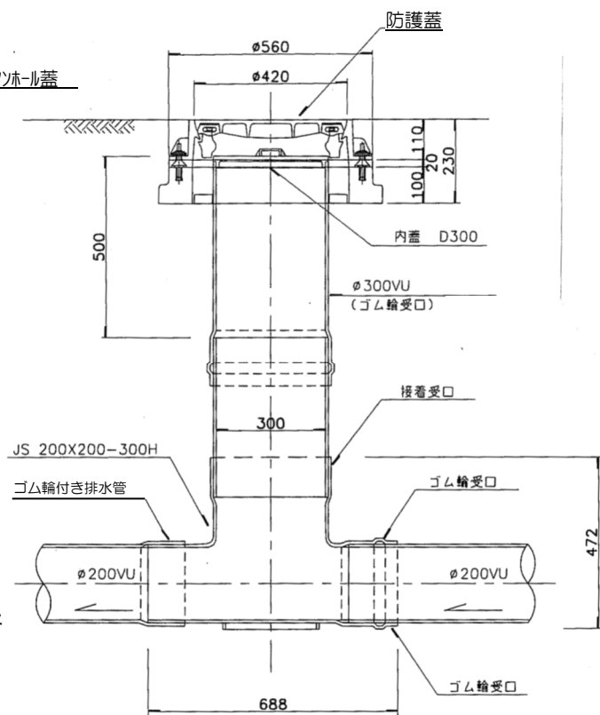
図3-6 小口径マンホール標準図 (本管φ200、立上管φ300の場合)
