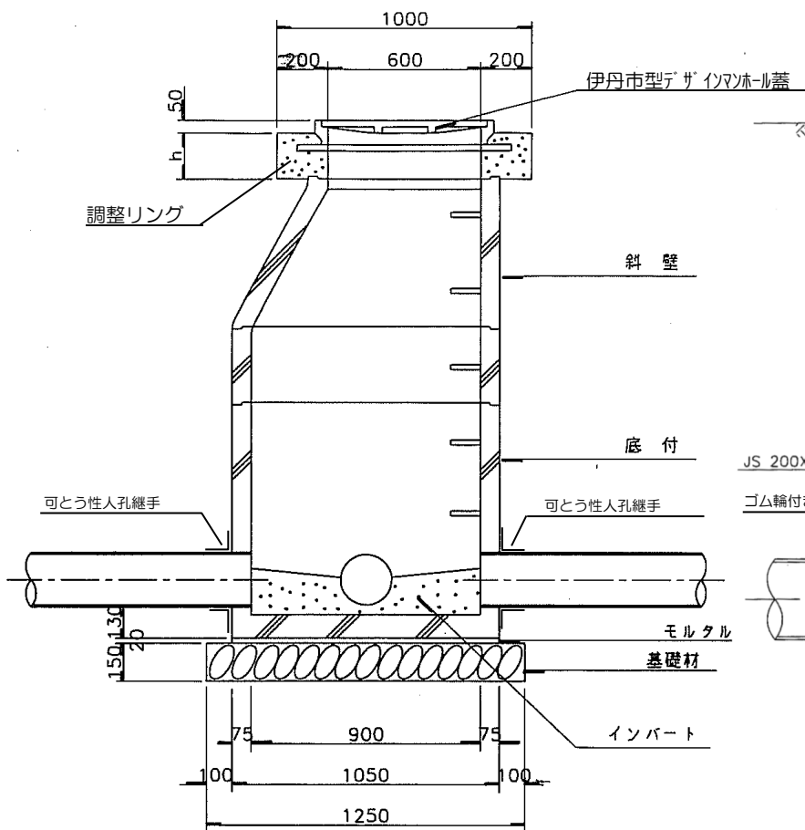
図3-6 小口径マンホール標準図 (本管φ200、立上管φ300の場合)
